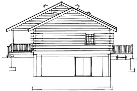
RIGHT ELEVATION
