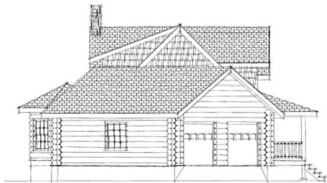
Right Elevation
