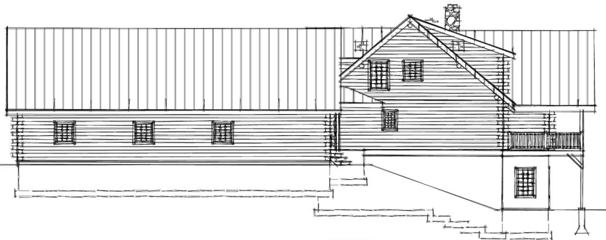
RIGHT ELEVATION
